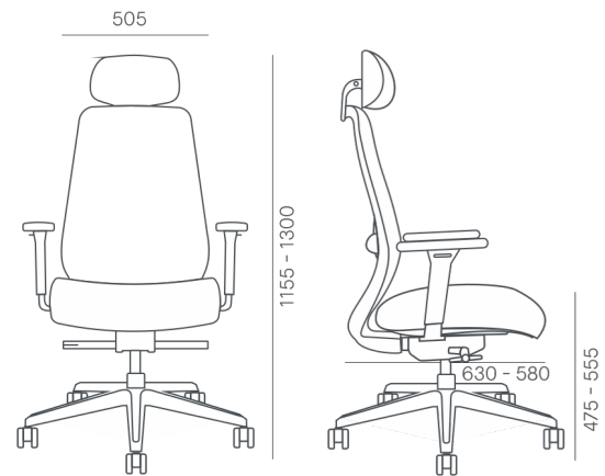
DIMENSIONES
